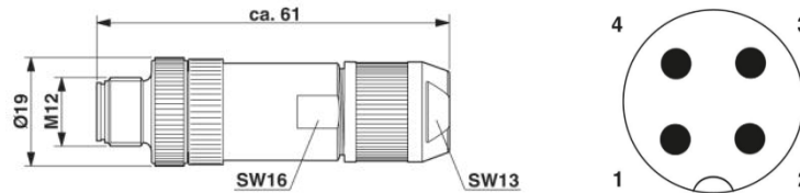
Bild 36: Stecker M12 x 1 gerade, geschirmt ; Polbild Stecker M12, 4-polig, A-kodiert, Ansicht Stiftseite.
