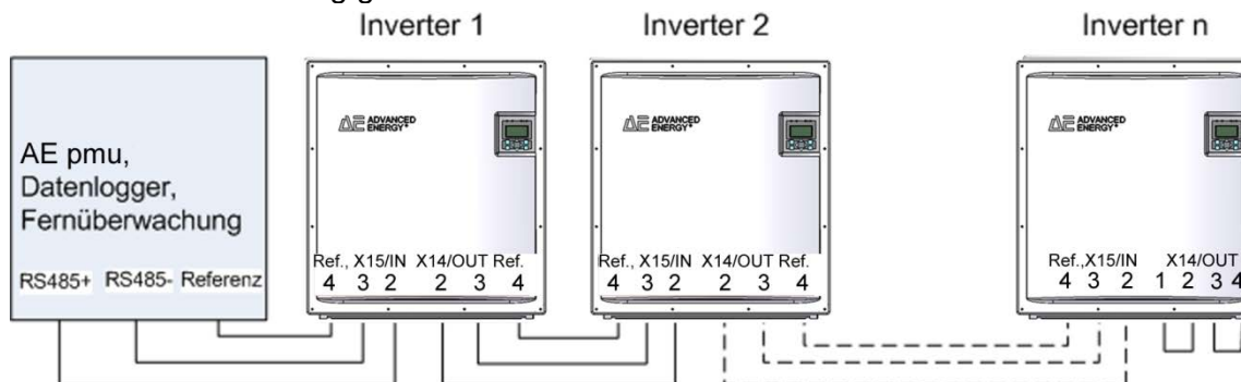
Bild 35: Standardschnittstelle
