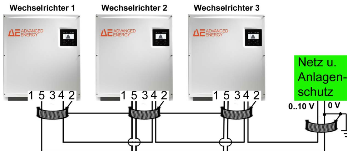
Bild 41: Schematische Erläuterung Standard-Konfiguration
