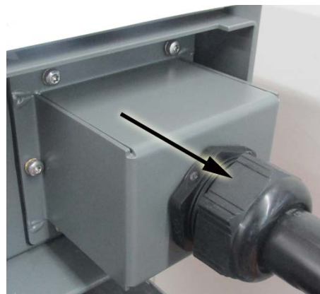
Bild 22: AC-Anschlussgehäuse festschrauben
