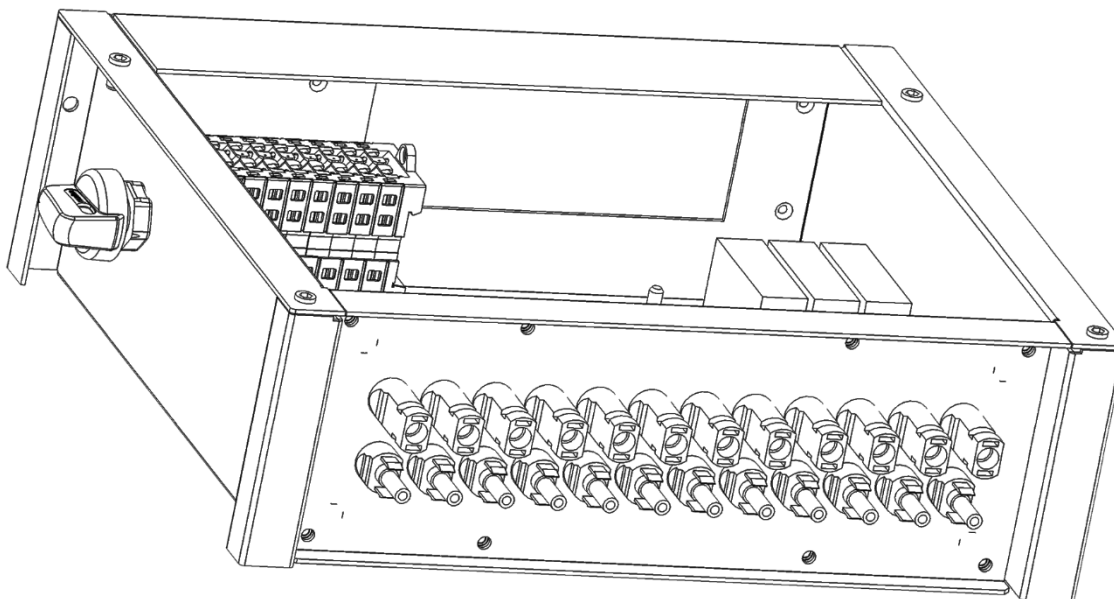
Bild 42: ConnectionBox mit Ein/Aus Schalter links und 12 DC-Anschlüssen
