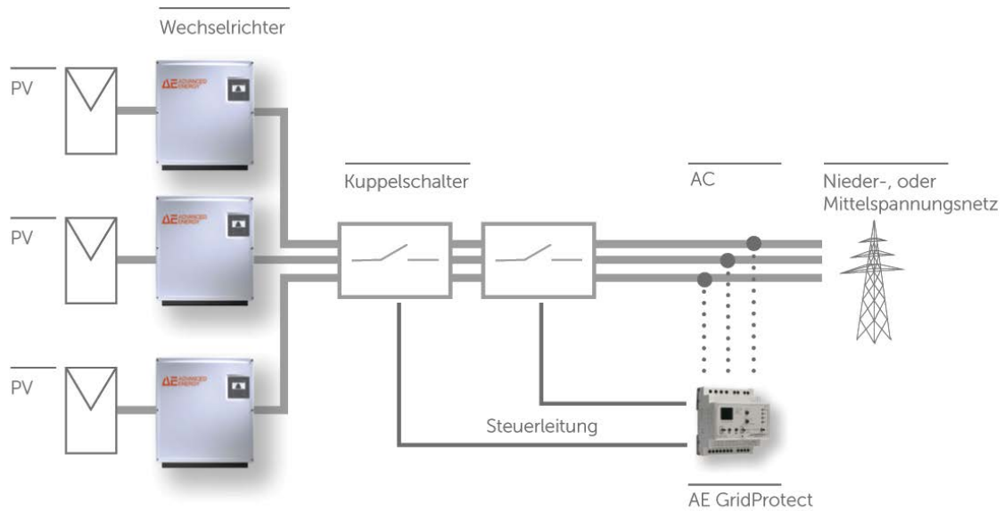
Bild 40: Beispiel zentraler Netz- und Anlagenschutz mit externen Kuppelschaltern
