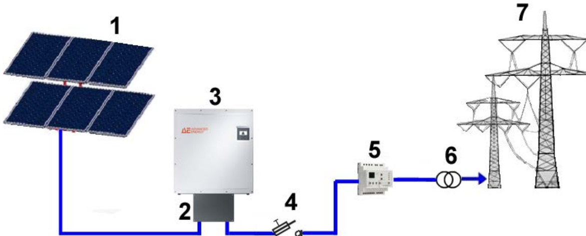
Bild 1: Funktionsprinzip einer netzgekoppelten PV-Anlage mit Photovoltaik-Wechselrichter REFUsof®
