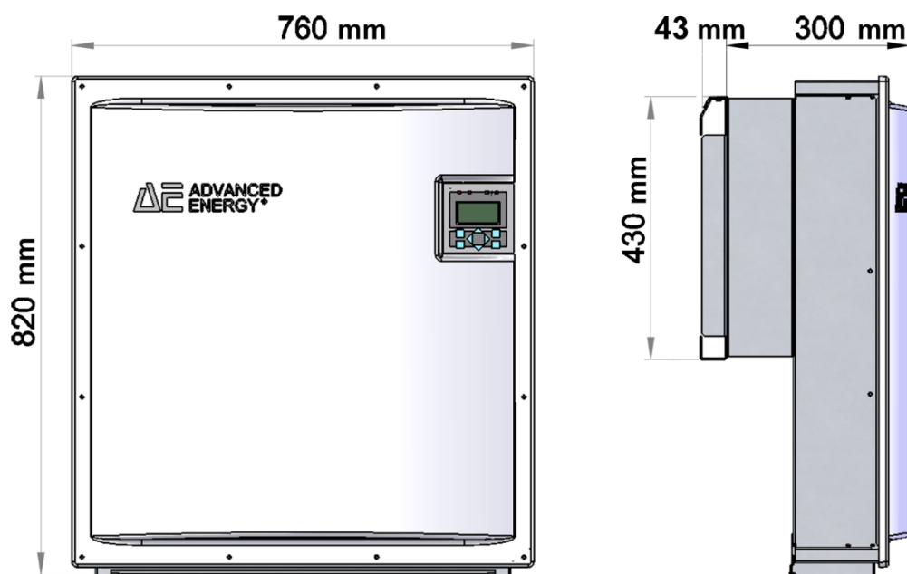
Bild 3: Gehäusemaße
