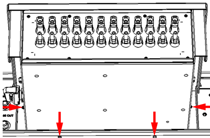
Bild 29: Lage der Befestigungsbohrungen
