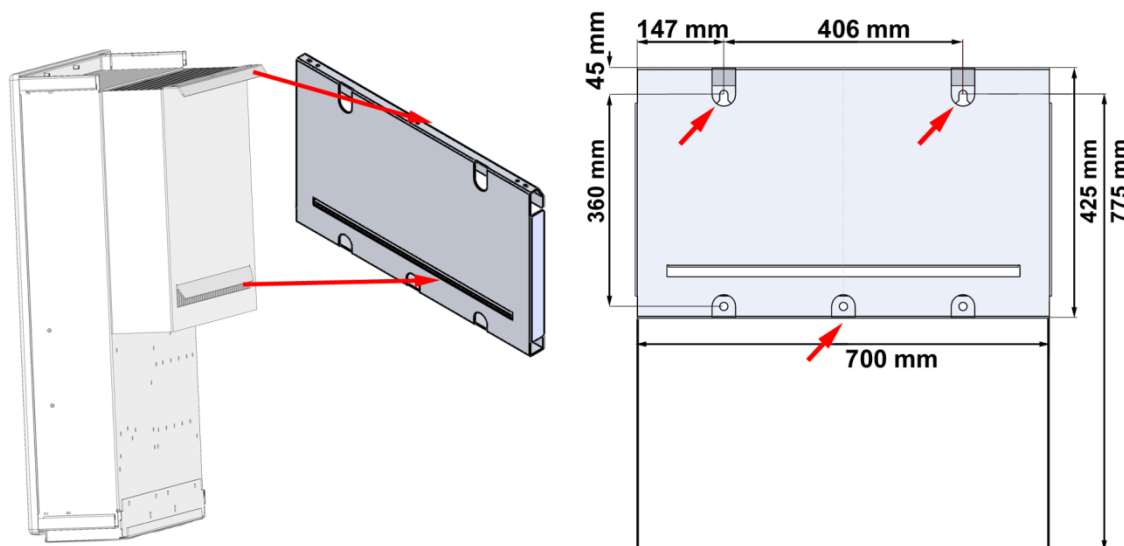
Bild 13: Gerätemontage
