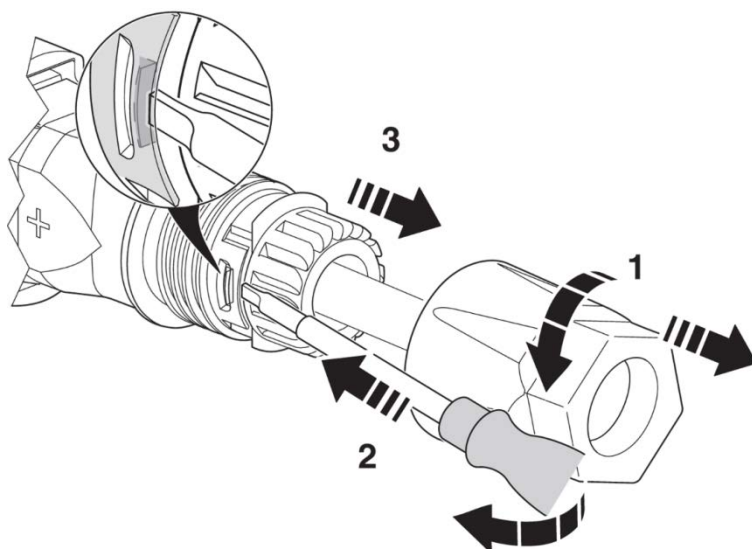
Bild 18: Kabel lösen
