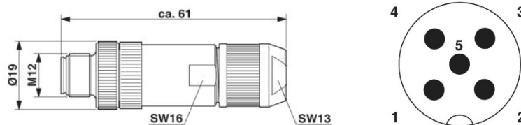
Bild 22: Stecker M12 x 1 gerade, geschirmt; Polbild Stecker M12, 5-polig, A-kodiert, Ansicht Stiftseite, PHOENIX CONTACT Bezeichnung: SACC-M12MS-5SC SH
