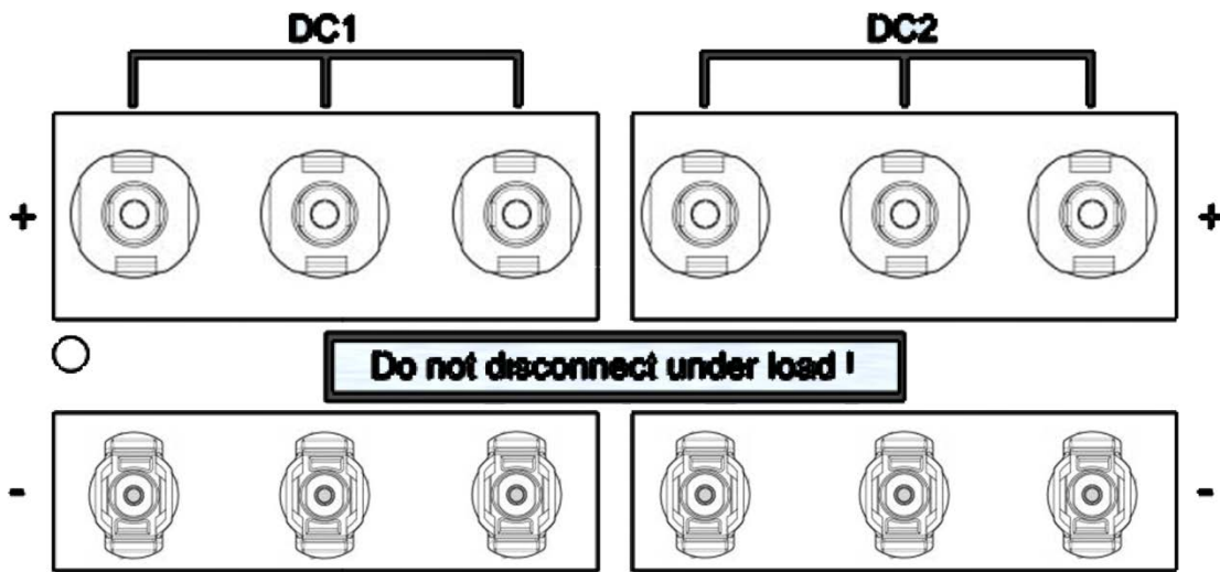
Bild 4: DC-Anschlussbereich
