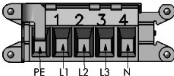
Bild 11: Netzanschluss
