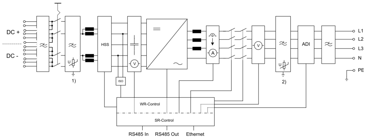
Bild 3: Blockschaltbild 3TL 8 ... 23
