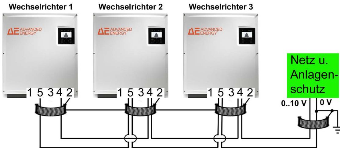
Bild 27: Schematische Erläuterung Standard-Konfiguration
