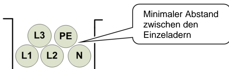
Bild 15: Kabelverlegung
