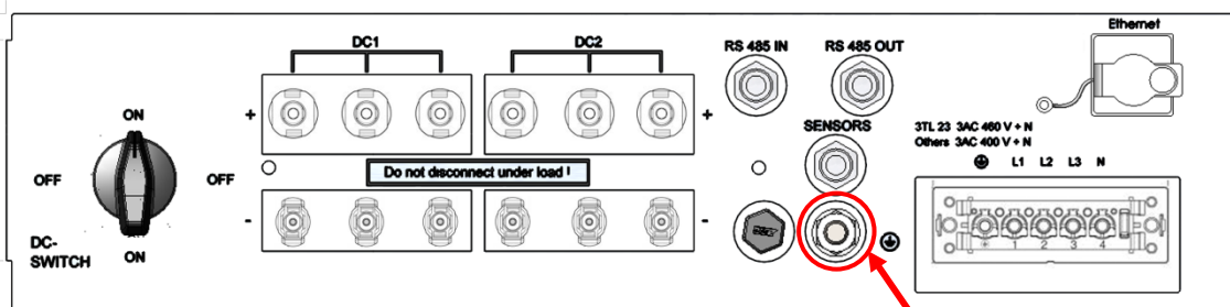
Bild 10: Erdungsbolzen
