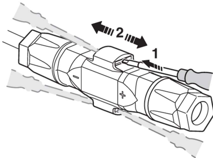
Bild 17: Steckverbinder trennen
