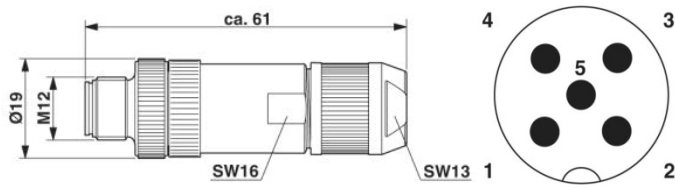
Bild 26: Sensorstecker M12 x 1 gerade, geschirmt; Polbild Sensorstecker M12, 5-polig, A-kodiert, Ansicht Stiftseite, Phoenix Bezeichnung: SACC-M12MS-5SC SH
