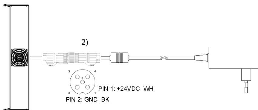
Bild 31: AE Powercap mit Steckernetzteil
