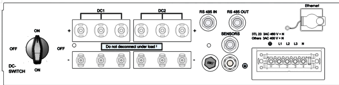
Bild 9: Geräteanschlüsse 3TL 8 ... 23
