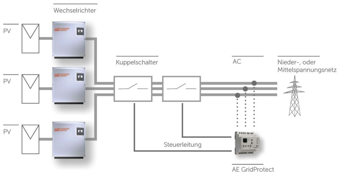
Bild 24: Beispiel zentraler Netz- und Anlagenschutz mit externen Kuppelschaltern
