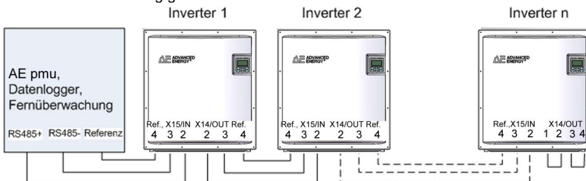
Bild 19: Standardschnittstelle
