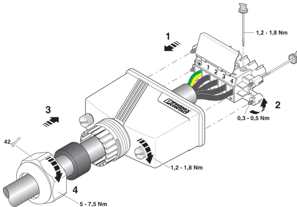
Bild 13: Stecker verschrauben
