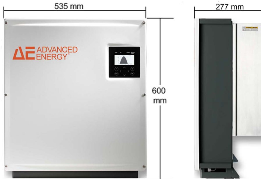
Bild 2: Gehäusemaße
