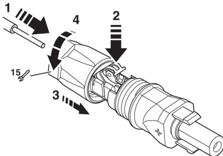
Bild 16: Kabel anschließen
