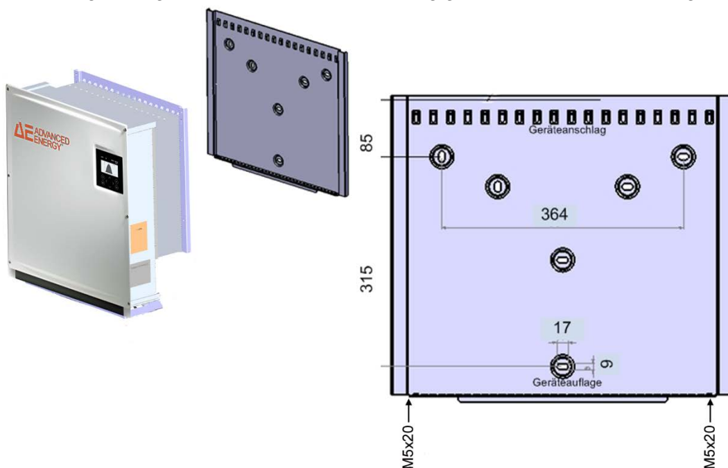
Bild 8: Gerätemontage
