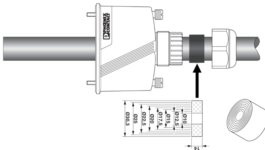
Bild 14: Durchmesser
