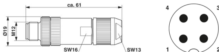
Bild 20: Stecker M12 x 1 gerade, geschirmt ; Polbild Stecker M12, 4-polig, A-kodiert, Ansicht Stiftseite.
