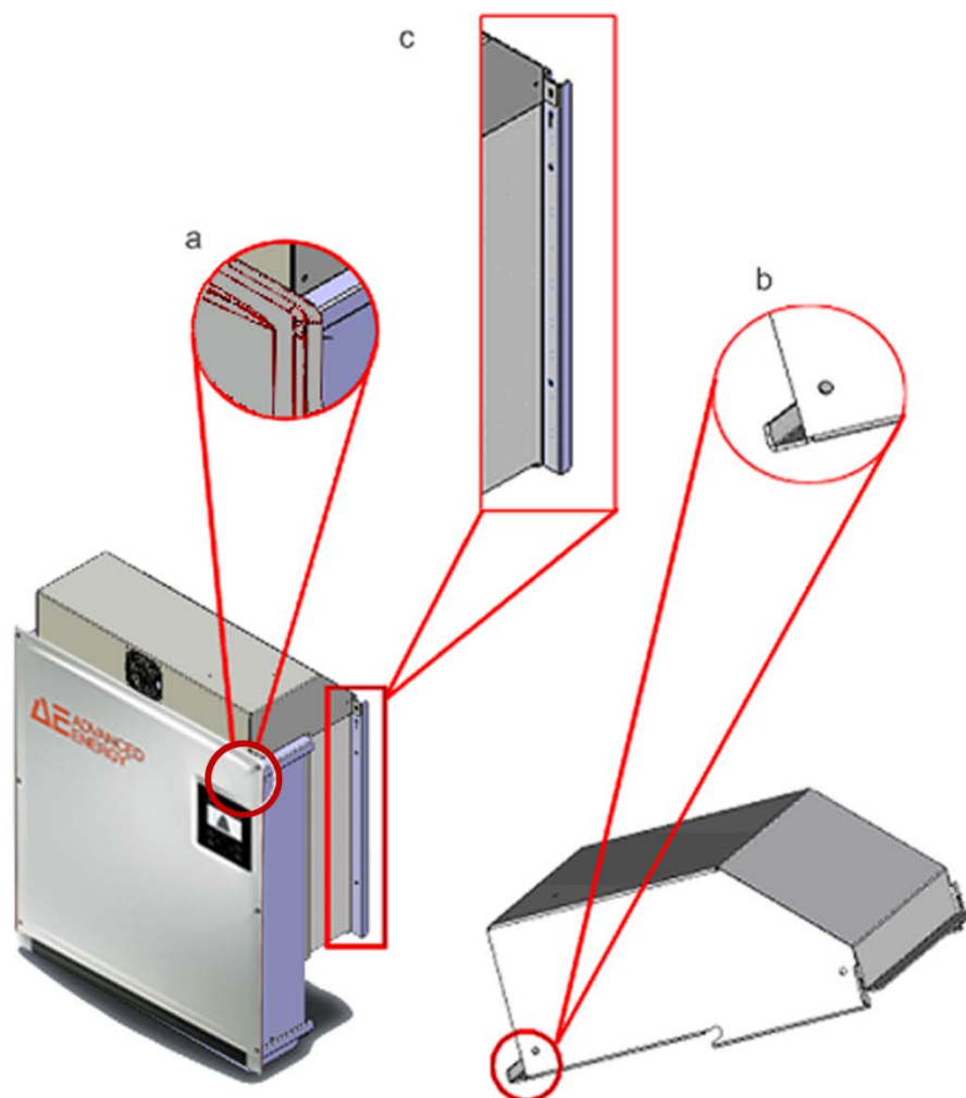
Bild 28: AE Powercap
