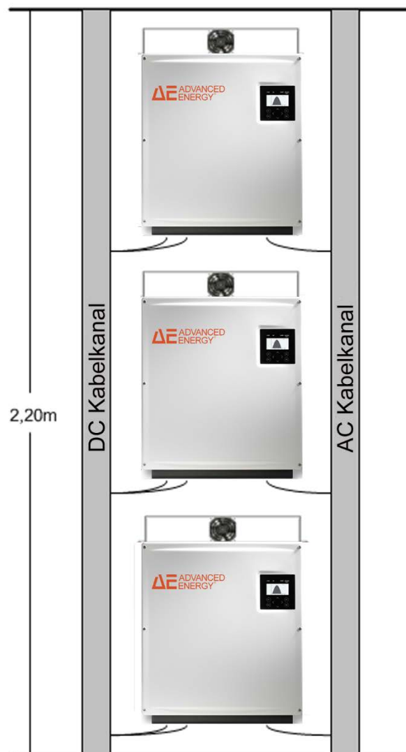
Bild 29: Montage AE Powercap
